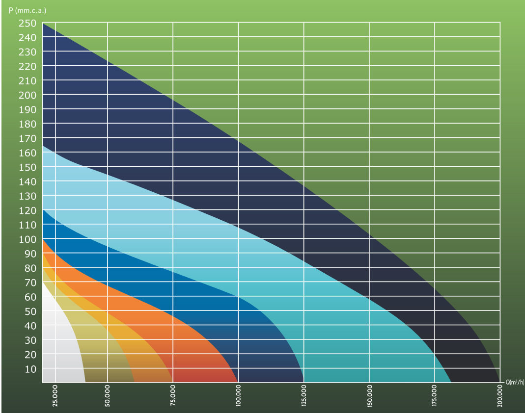
Gráfico de Performance - Vazão (m³/h) X Pressão Disponível (mm.c.a.)
